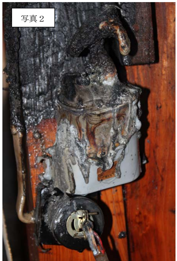
低圧進相コンデンサの拡大写真。
