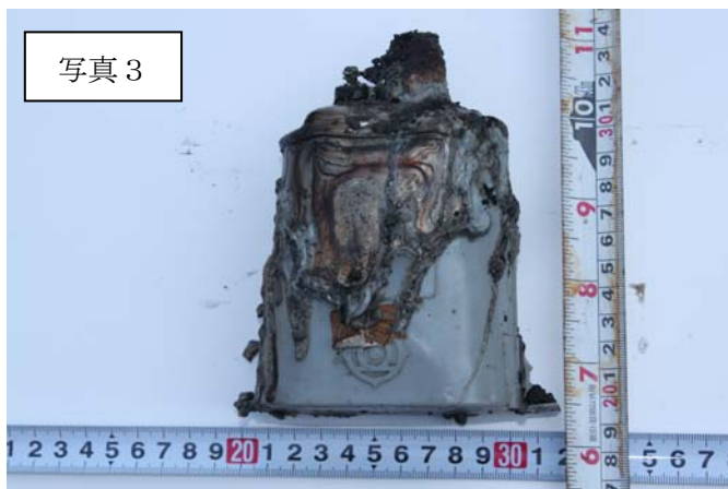
低圧進相コンデンサの拡大写真。
