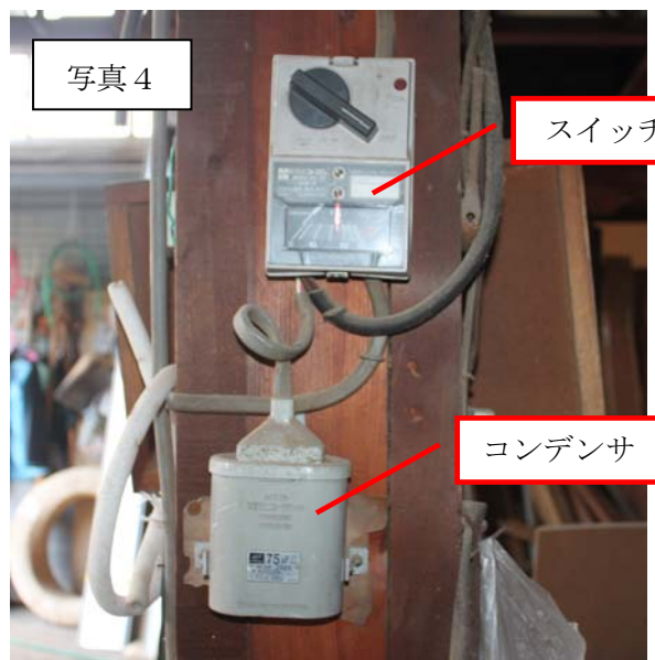
低圧進相コンデンサの設置例。
